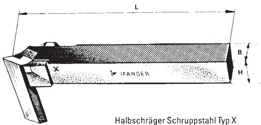
Halbschräger Schruppstahl Typ X
